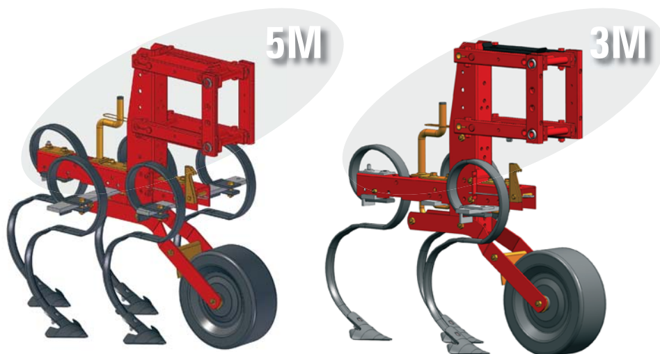
Elemento standard a 5 molle flessibili Standard unit with 5 flexible tines Standardelement mit 5 Zinken Стандартный агрегат с 5 гибкими пружинами
